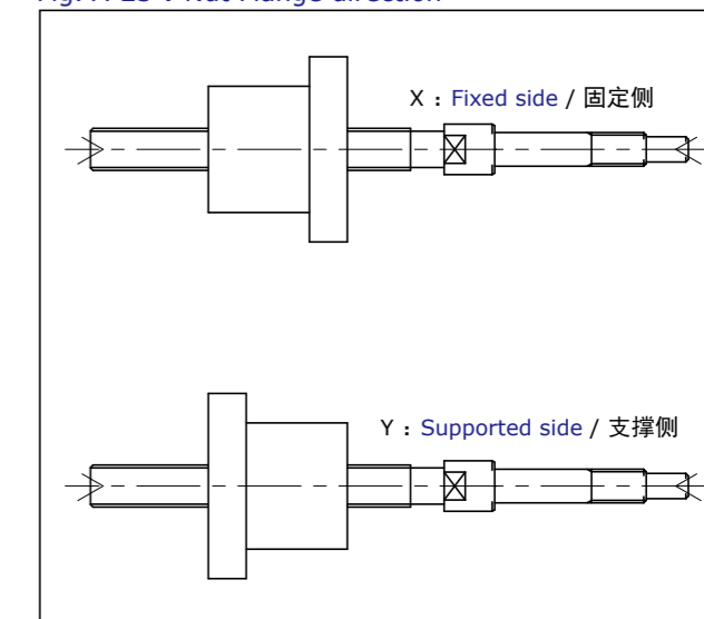
图A-23 : 螺母法兰朝向 Fig. A-23 : Nut Flange direction
